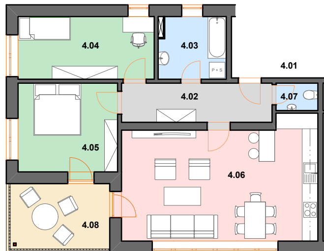
PŮDORYS BYTU
